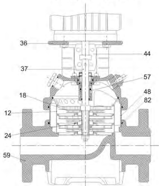
AV-1,3,5,10,15,20
