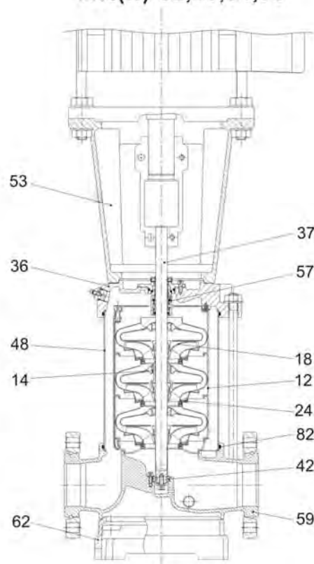
AVI(N)-32,45,64,90
