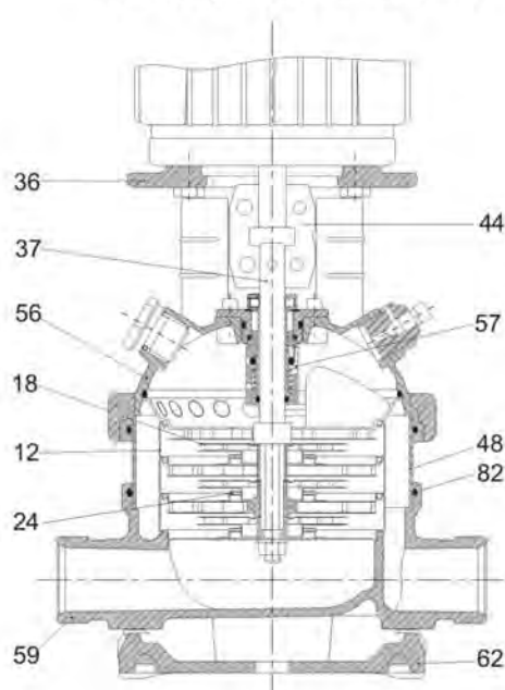
AVI(N)-1,3,5,10,15,20
