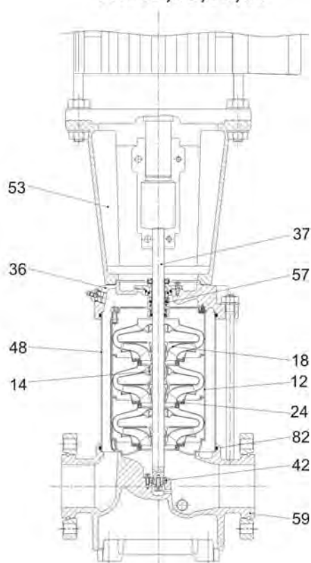
AV-32,45,64,90
